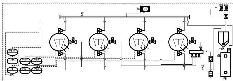
Schéma základního vybavení (systém nízkého tlaku oleje):
