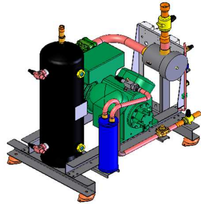
Schéma základního vybavení:
