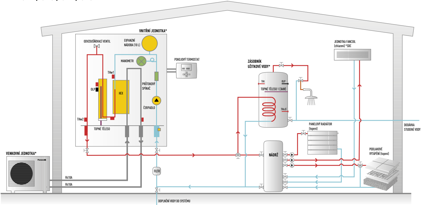
Schematický náčrtek
