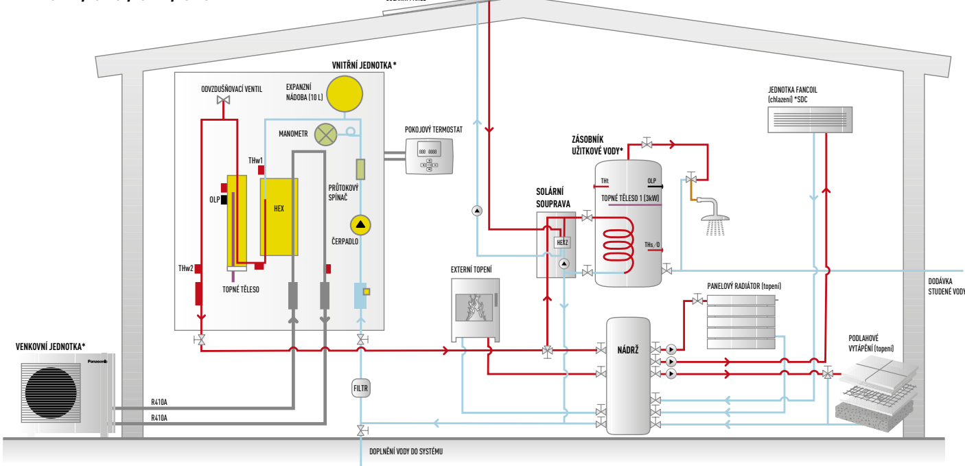
Schematický náčrtek
