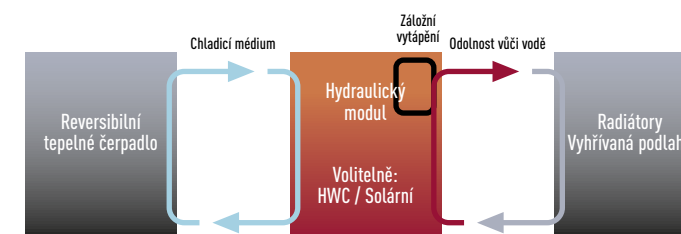
Příklad : s rozdělným systémem
